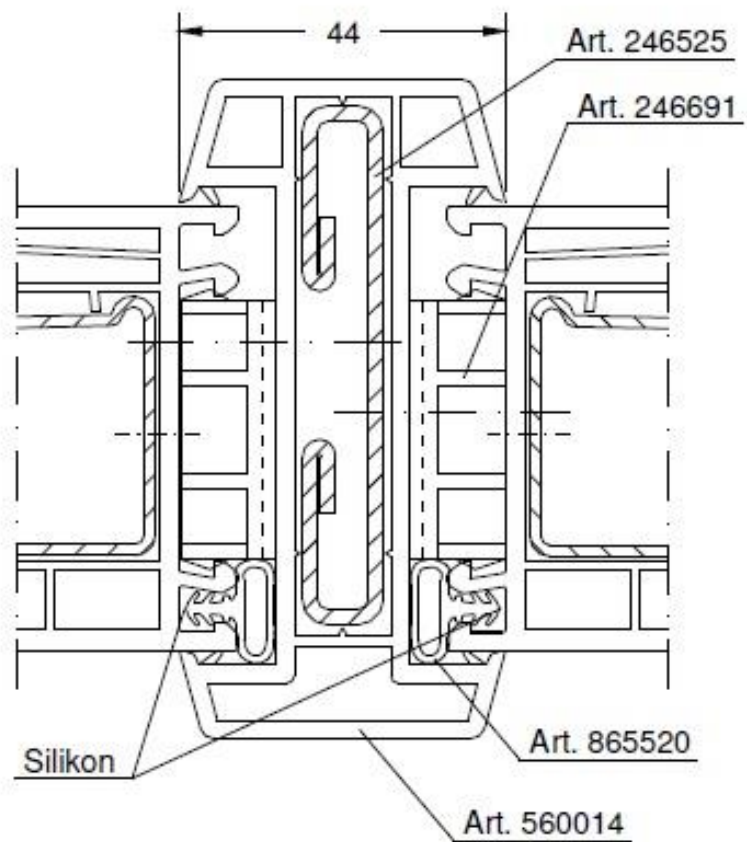
Connettore affacciato da 18 mm
